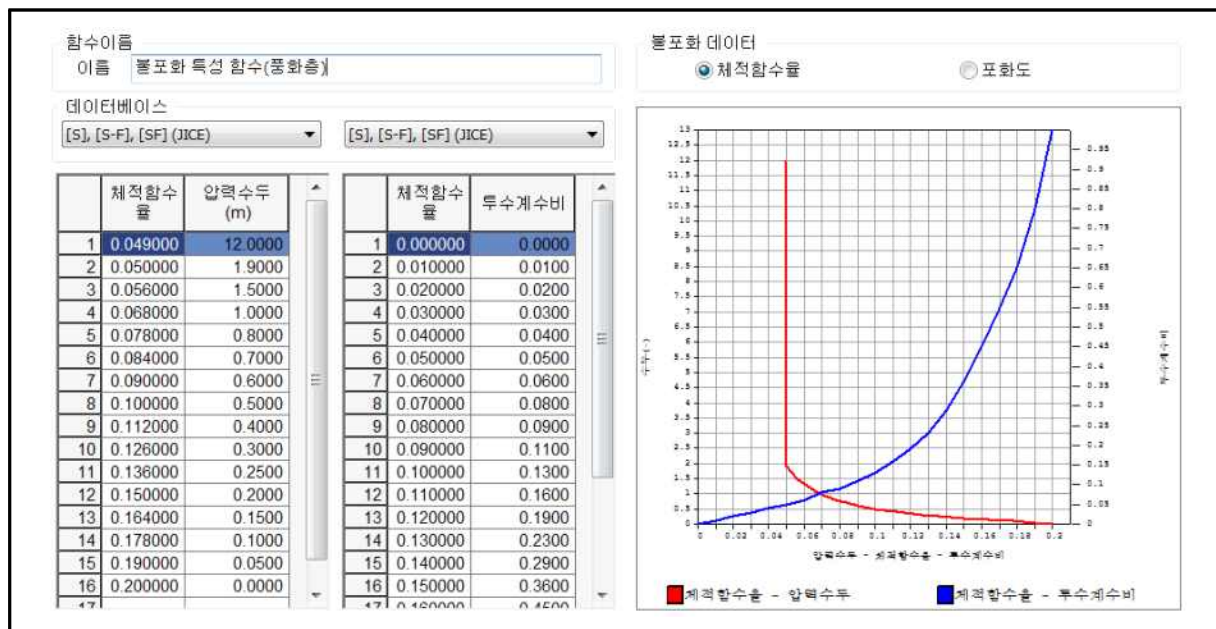
【그림 23.15】 압력수두-체적함수율(포화도)-투수계수비 함수
