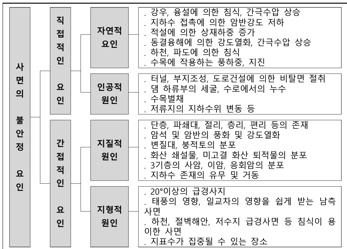
【그림 23.6】 구조안전성능 평가과정
